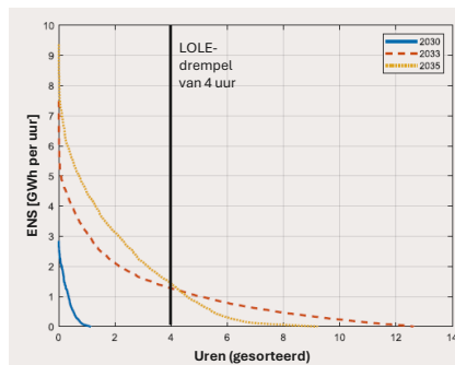
Figuur 5: Duurcurves voor Energy Not Served (ENS). Bron: Aangepast van TenneT, Monitor Leveringszekerheid 2025, figuur 4-4. 1
