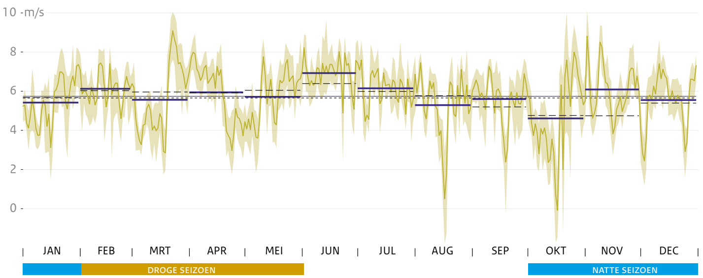
Windsnelheid Bonaire
